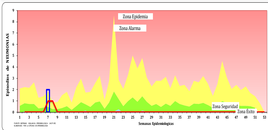
CANAL ENDEMICO DE NEUMONIAS POR SEMANAS EPIDEMIOLOGICAS RED HUAROCHIRI A LA S.E 14 AÑO 2023
